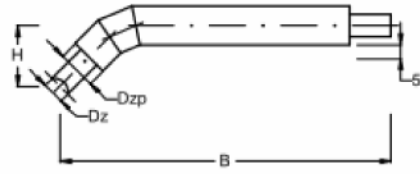
Kolano odgałęźne
