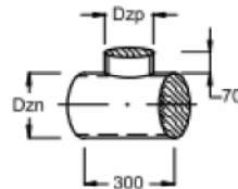
Trójnik TPE
